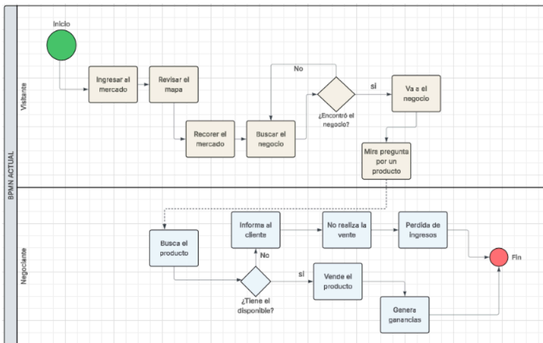
Figura 68 BPMN
